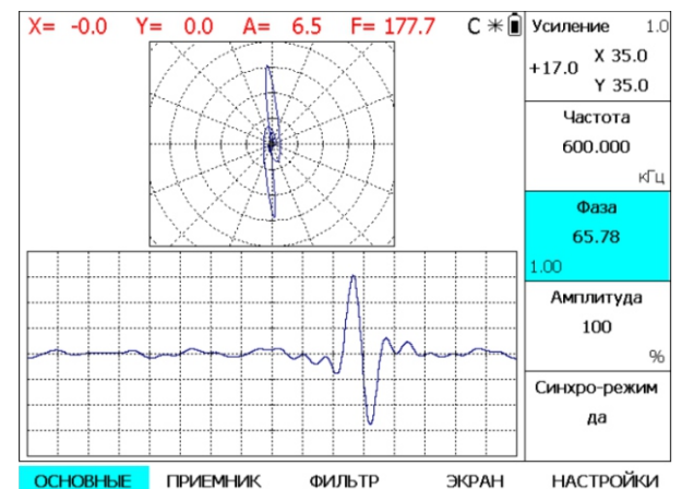
Изображение экрана после настройки преобразователя RVS-15 по контрольному дефекту
