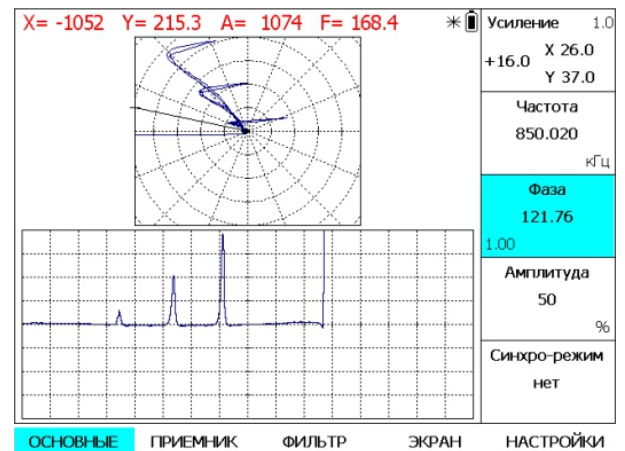
Результат сканирования образца ВСО-2 из алюминия после настройки.
